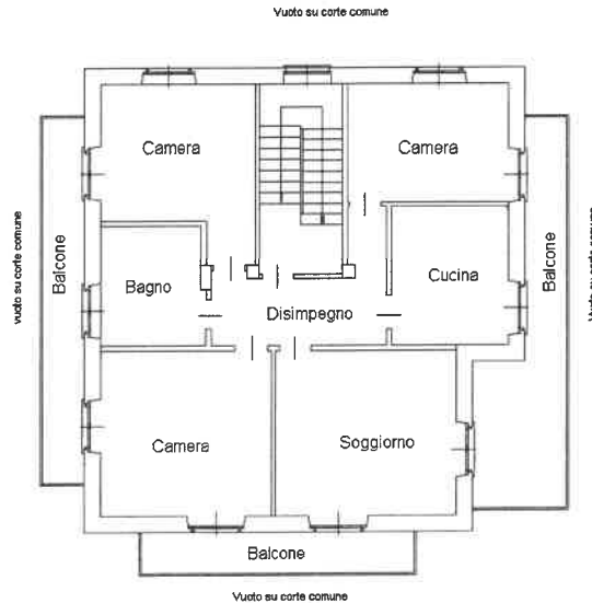
PIANO PRIMO h=2,80 m
