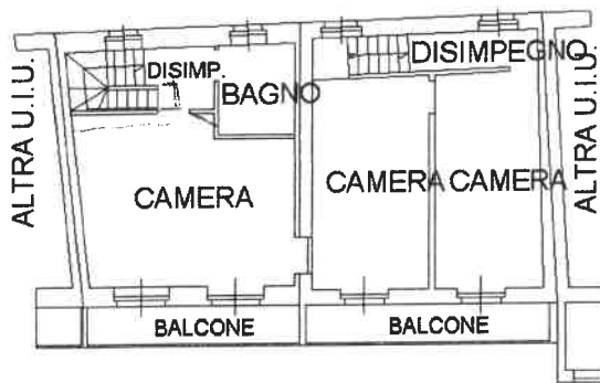
PIANO PRIMO h m. 2,70
